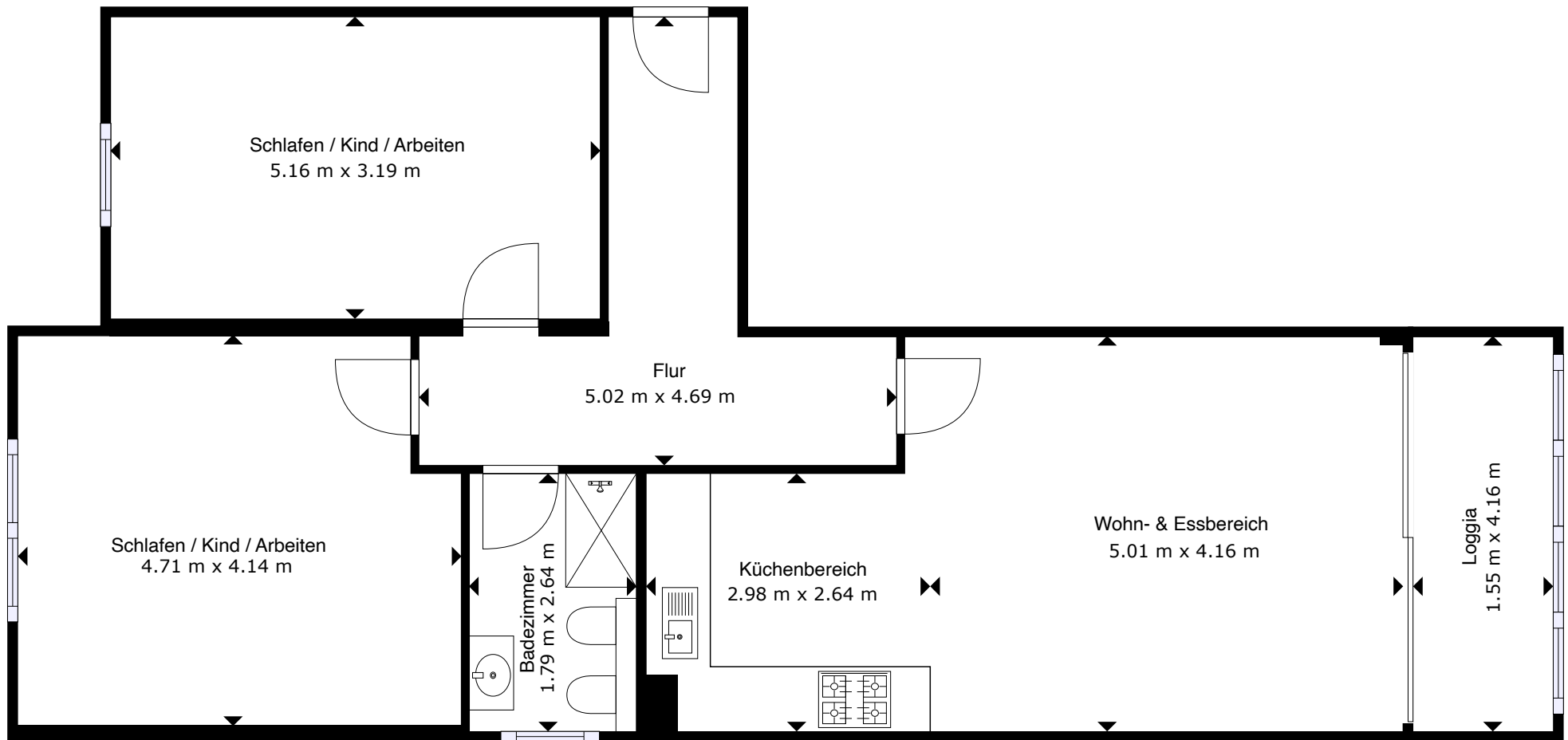
1. Obergeschoss
